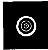
انعراج الضوء خلال ثقب صغير جداً
